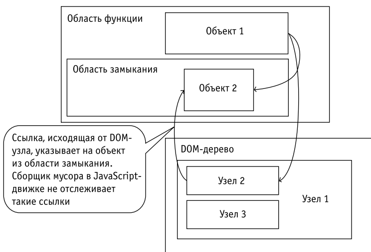
Рис. 7.4. Циклические ссылки с самозамыканием
