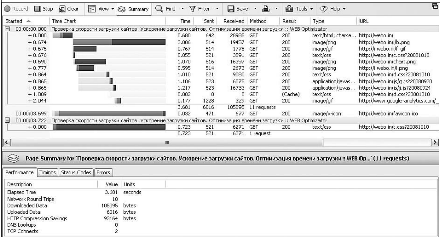
Рис. 8.6. Результаты анализа загрузки сайта в HttpWatch
