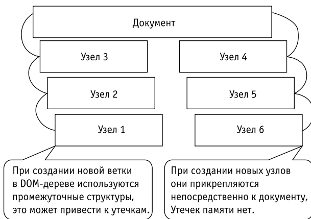
Рис. 7.5. Утечки, связанные с порядком добавления DOM-элементов
