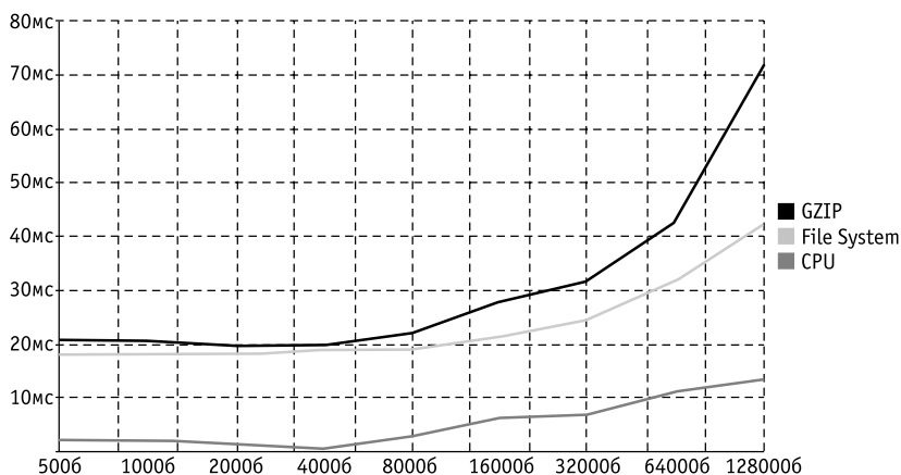
Рис. 2.2. График издержек на gzip-сжатие и работу с файловой системой
