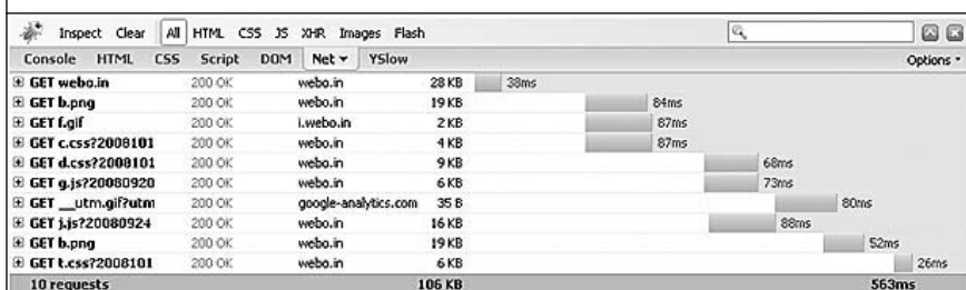
Рис. 8.3. Результаты анализа загрузки сайта в Firebug Net Panel
