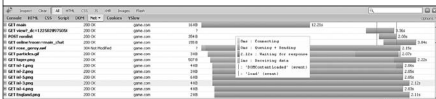
Рис. 8.2. Результаты анализа загрузки сайта в Firebug Net Panel 1.4a1
