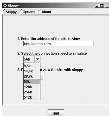
Рис. 8.9. Настройки Sloppy для тестирования загрузки сайта на медленном канале
