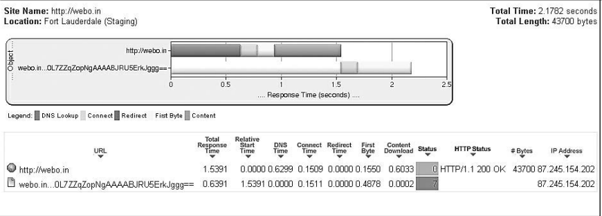
Рис. 8.13. Результаты анализа загрузки сайта в www.alertsite.com/cgi-bin/tsite3.pl
