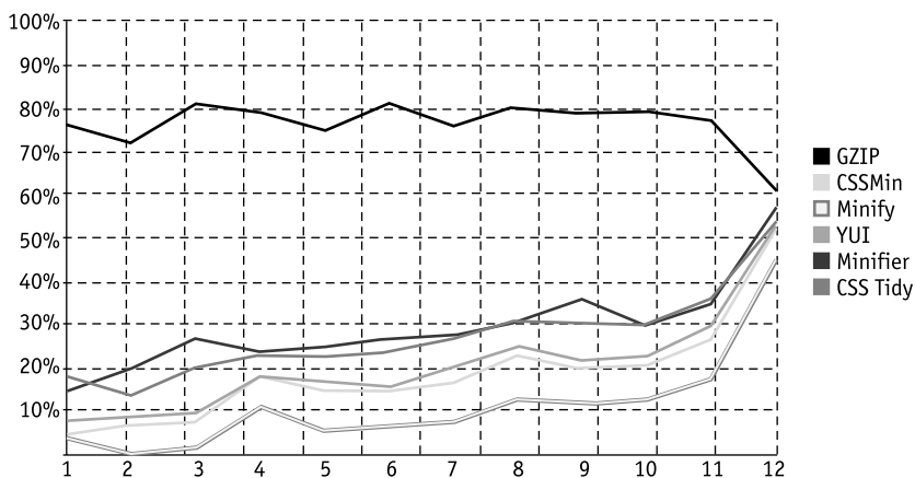
Рис. 2.7. Эффективность различных инструментов для минимизации CSS-файлов по сравнению с gzip
