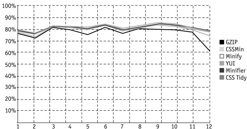
Рис. 2.8. Эффективность различных инструментов для минимизации CSS-файлов вместе с дополнительным архивированием по сравнению с gzip
