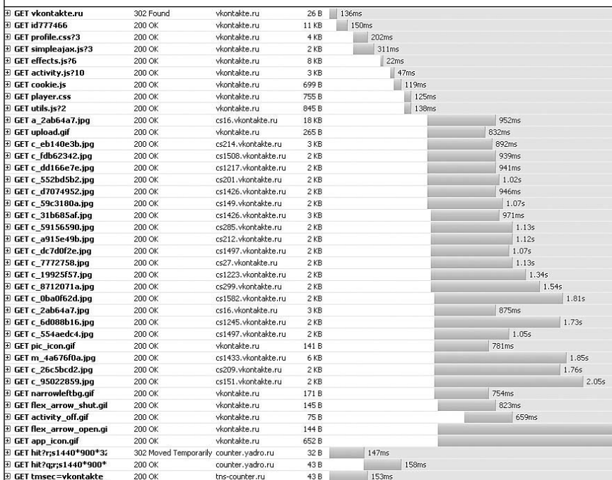
Рис. 8.18. Результаты анализа загрузки внутренней страницы сайта vkontakte.ru
