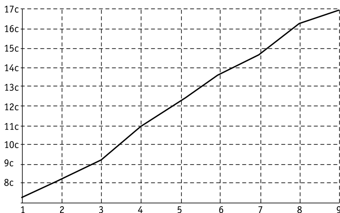
Рис. 2.5. Зависимость издержек на gzip от степени сжатия
