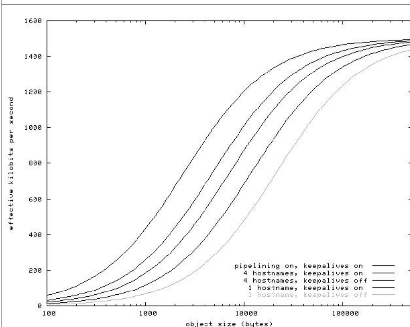
Рис. 5.4. Влияние HTTP-конвейера и постоянного соединения на скорость передачи данных. Источник: www.die.net
