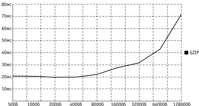
Рис. 2.1. График издержек на gzip-сжатие от размера файла
