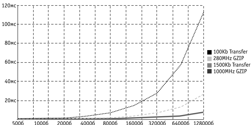
Рис. 2.4. Накладные издержки на сжатие и передачу информации для 100 Кб и 1500 Кб и 280 МГц и 1000 МГц
