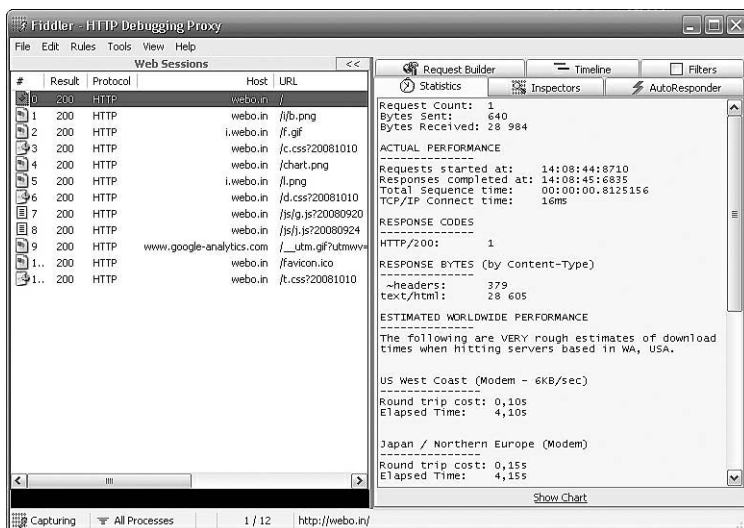
Рис. 8.7. Результаты анализа загрузки сайта в Fiddler
