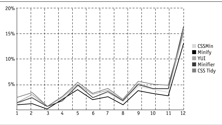
Рис. 2.9. Эффективность различных инструментов для минимизации CSS-файлов вместе с дополнительным архивированием (увеличенный масштаб)
