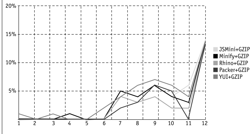
Рис. 2.12. Эффективность различных инструментов для минимизации JavaScript-файлов вместе с дополнительным архивированием (увеличенный масштаб)
