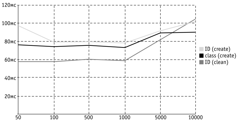
Рис. 6.1. Время создания документа (средневзвешено по всем браузерам)
