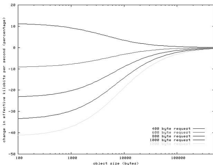
Рис. 5.6. Влияние заголовков на эффективную пропускную способность канала. Источник: www.die.net
