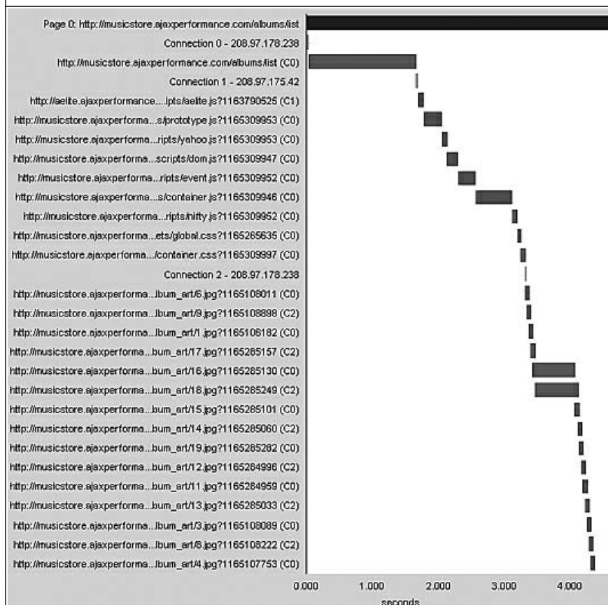
Рис. 5.1. Загрузка изображений при двух соединениях.
