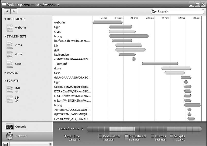
Рис. 8.5. Результаты анализа загрузки сайта в Web Inspector
