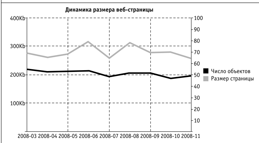
Рис. 1.1. Тенденция изменения размера страницы и числа объектов для сайтов, проверяемых через Web Optimizator в 2008 году
