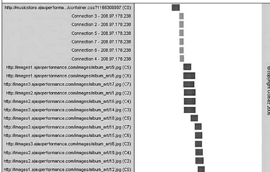
Рис. 5.2. Загрузка при шести соединениях. Источник: www.ajaxperformance.com
