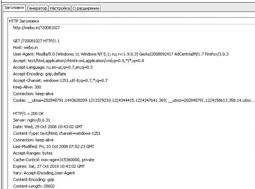
Рис. 8.8. Заголовки запроса и ответа в Live HTTP Headers для webco.in
