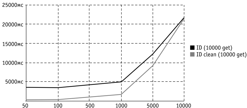
Рис. 6.2. Скорость выбора элемента (средневзвешено по всем браузерам)
