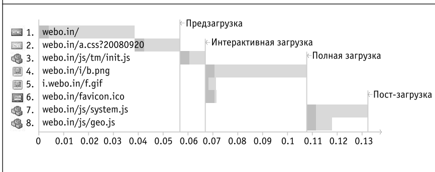
Рис. 1.2. Стадии загрузки страницы
