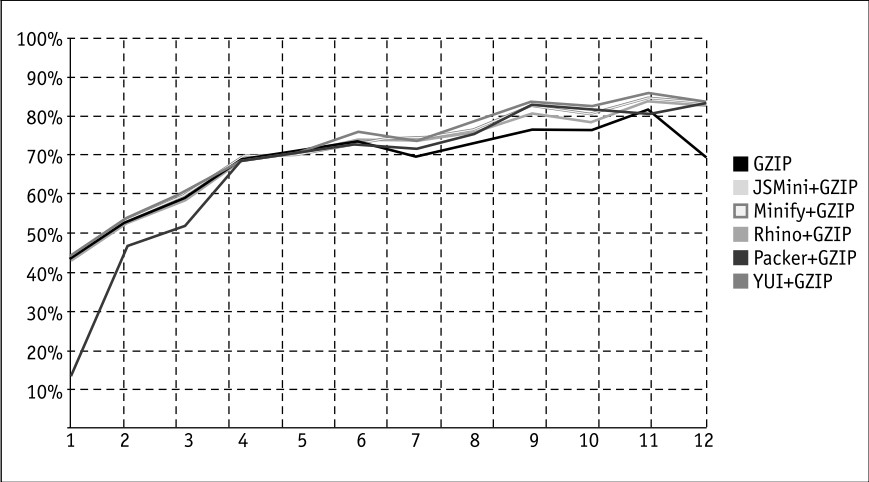
Рис. 2.11. Эффективность различных инструментов для минимизации JavaScript-файлов вместе с дополнительным архивированием по сравнению с gzip
