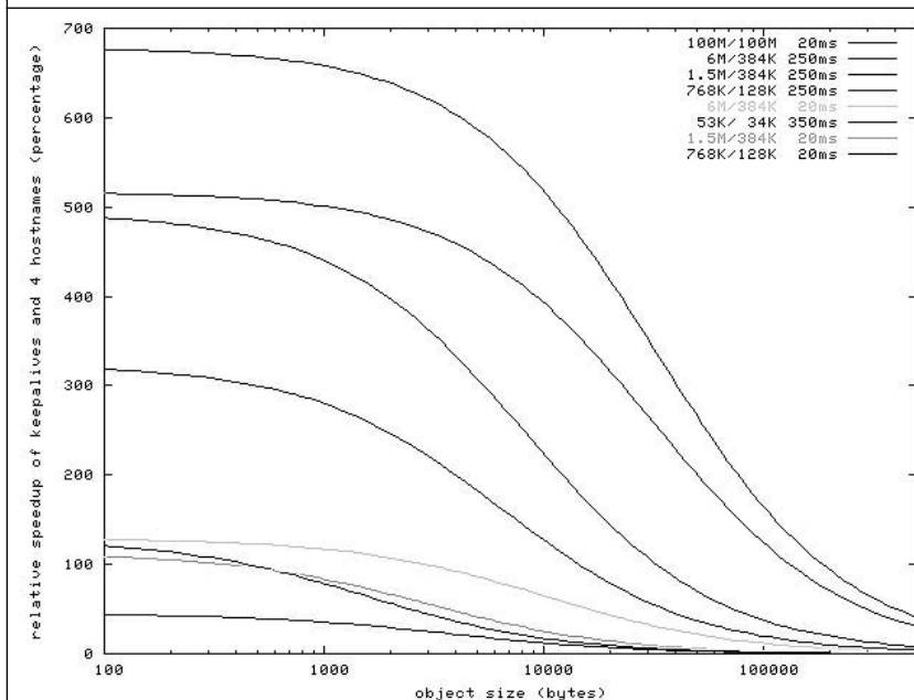
Рис. 5.5. Выигрыш при включении постоянного соединения и нескольких хостов для различных пользователей. Источник: www.die.net
