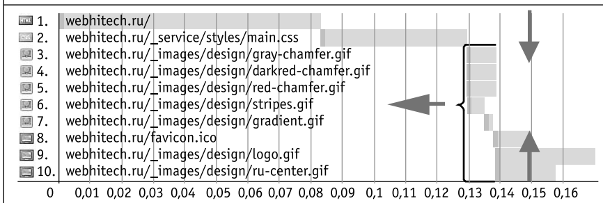
Рис. 5.7. Диаграмма загрузки (неизмененного) сайта WebHiTech.ru
